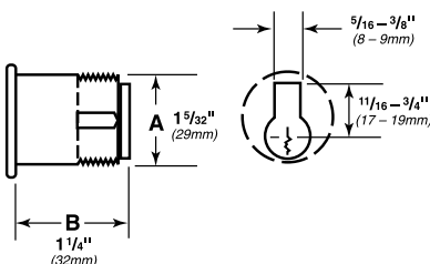
Mortise — 3215 (Schlage 20-001, L583-477 cam)
