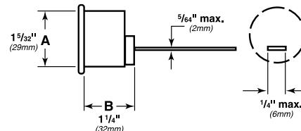
Rim — 3216 (Schlage 20-022)
